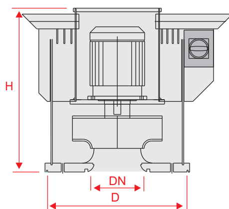
Roof Radial Fan
